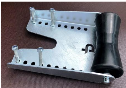
Kielrollenhalter Pongratz Gr. 1 für Quer- träger, feuerverzinkt. Höhe Befestigungsprofil ca. 290mm, Breite ca. 220mm Lochgrösse 11mm. Inkl. 2 Befestigungs U-Bügel M10, Abstand Schraubenmitte ca. 75mm Schraubenlänge ca. 65mm Miet-Lift Art. Nr. 50234
