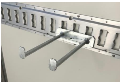
Doppelhaken / Werkzeughaken für Loch-/ Schlitzschiene Stahl feuerverzinkt. Abstand Mitte Haken 100mm, Hakenlänge 210mm Miet-Lift Art.Nr. 58195
